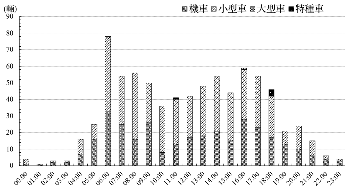
圖2.5-1 永樂路24小時單位車輛組織柱狀圖
