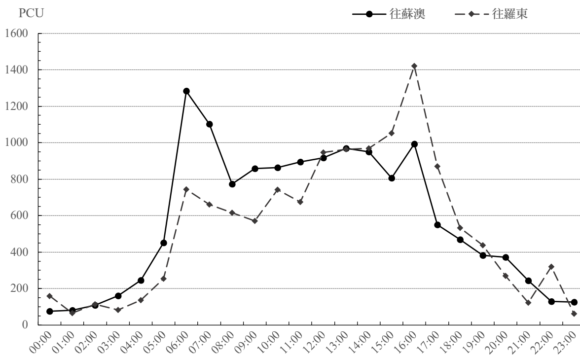
圖2.5-4 台九線24小時PCU變化圖
