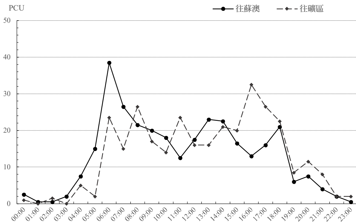
圖2.5-2 永樂路24小時PCU變化圖
