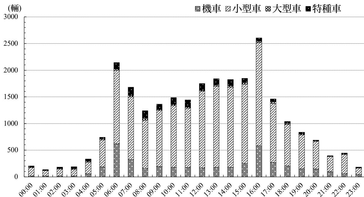
圖2.5-3 台九線24小時單位車輛組織柱狀圖
